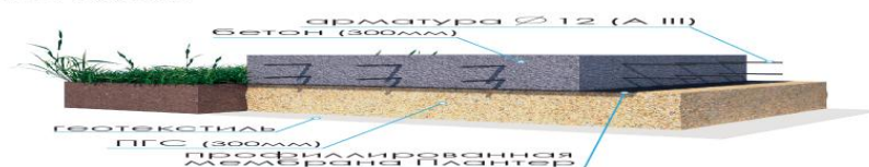
Монолитный фундамент плита 300мм
