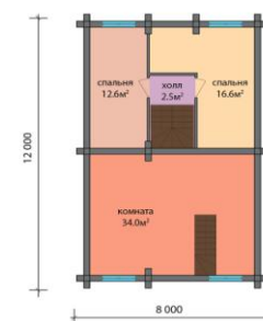
План 2 этажа
