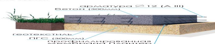
Монолитный фундамент плита 300мм
