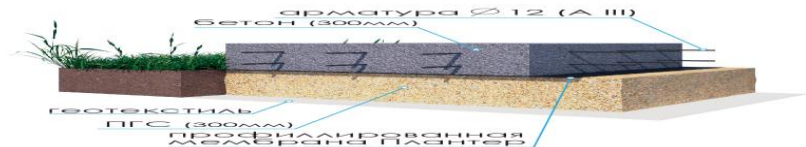
Монолитный фундамент плита 300мм
