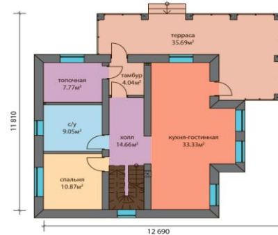
План 1 этажа
