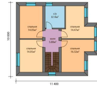
План 2 этажа
