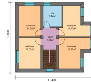
План 2 этажа
