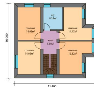
План 2 этажа
