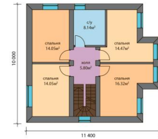
План 2 этажа
