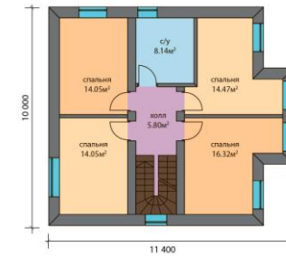
План 2 этажа
