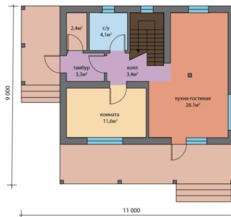
План 1 этажа
